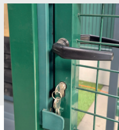
Serrure encastré Avec gâche en polyamide
